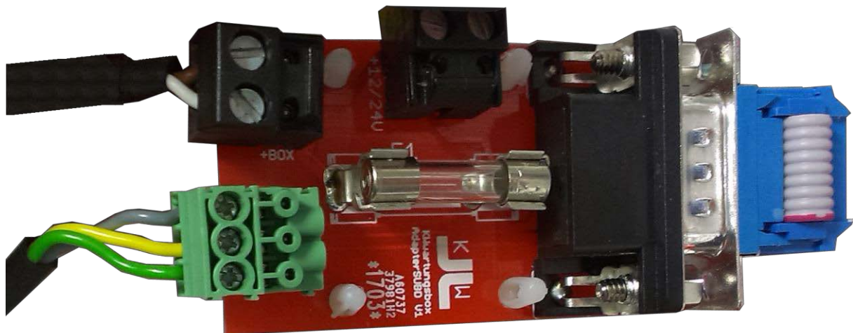
Abbildung 1- SUB-D Adapterplatine
