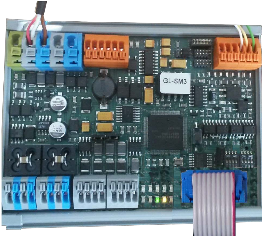
Abbildung 2- SM3 Redundanzmodul
